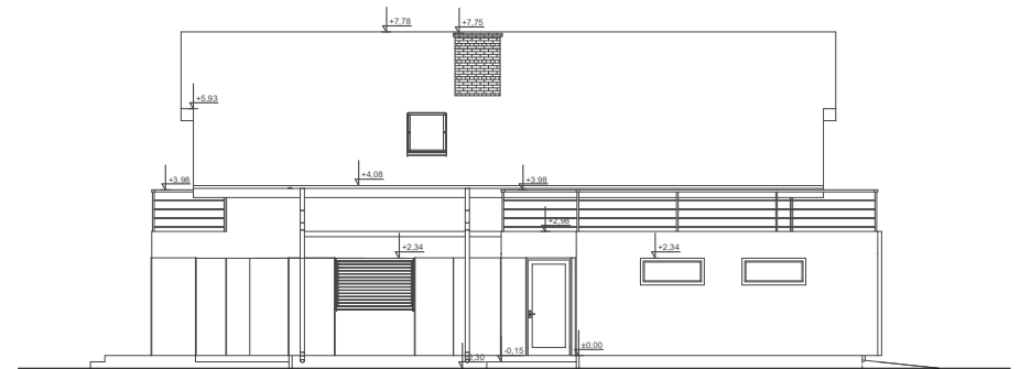
ELEWACJA BOK 1
