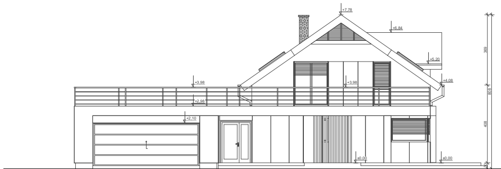
ELEWACJA FRONTOWA
