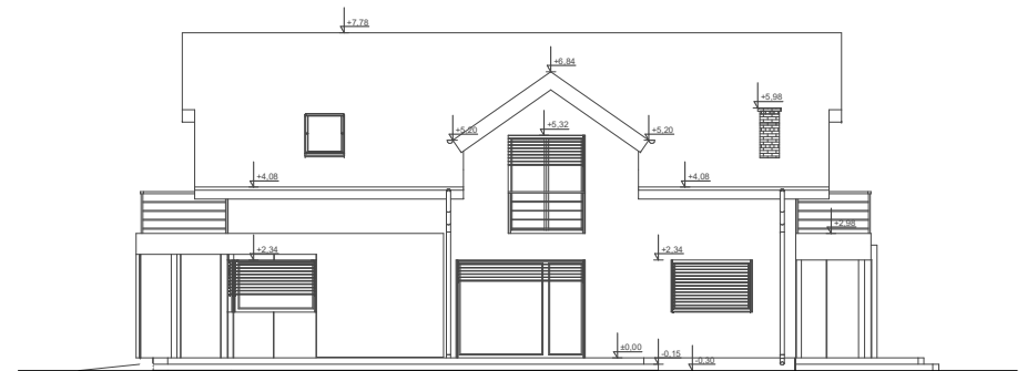
ELEWACJA BOK 2
