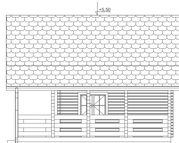
ELEWACJA BOK 2
