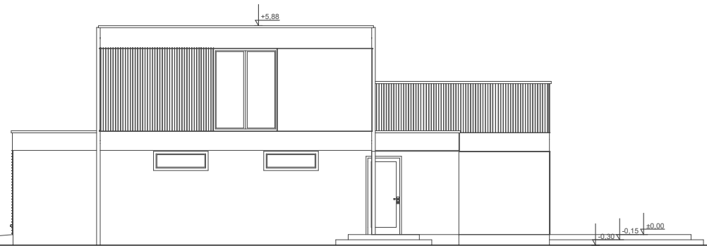
ELEWACJA BOK 2
