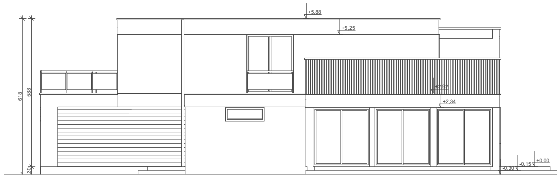
ELEWACJA OGRODOWA
