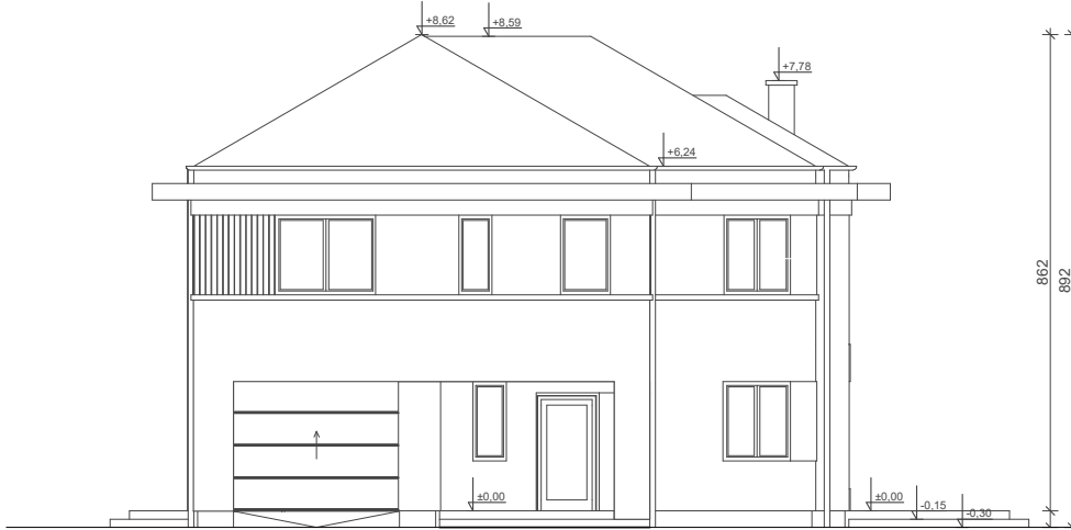
ELEWACJA FRONTOWA
