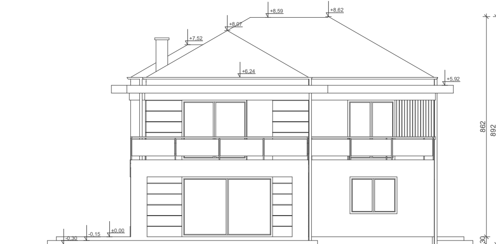
ELEWACJA OGRODOWA
