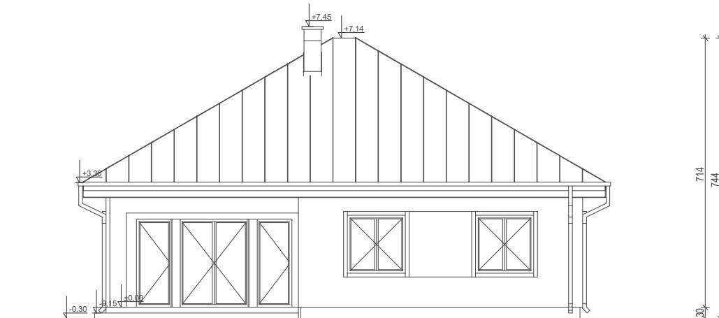
ELEWACJA OGRODOWA
