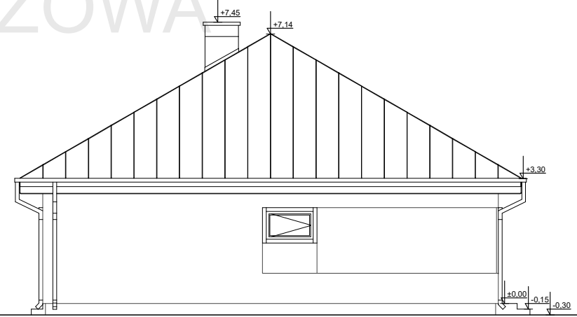
ELEWACJA BOK 1
