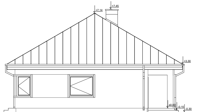
ELEWACJA BOK 2
