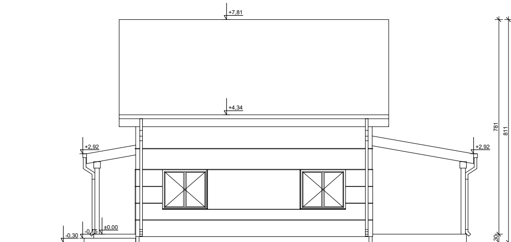
ELEWACJA OGRODOWA
