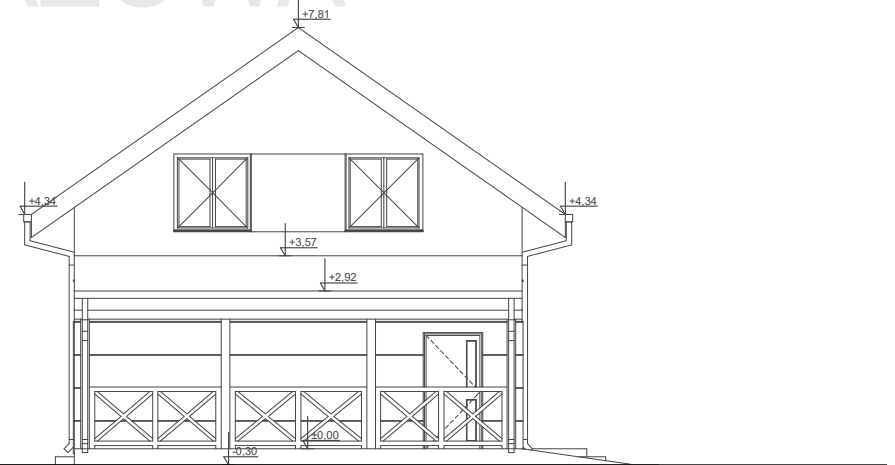
ELEWACJA BOK 1
