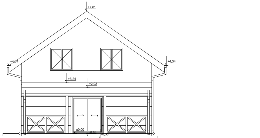
ELEWACJA BOK 2
