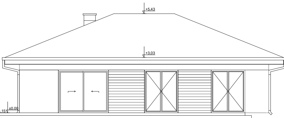
ELEWACJA OGRODOWA
