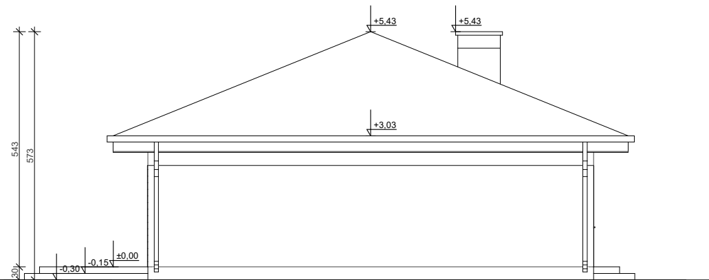
ELEWACJA BOK 1
