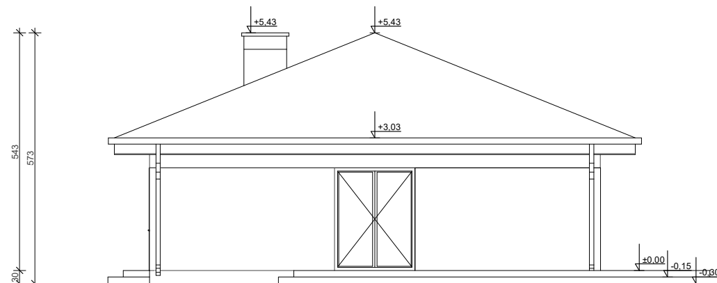
ELEWACJA BOK 2
