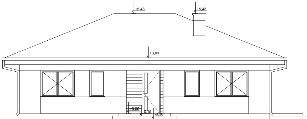
ELEWACJA FRONTOWA
