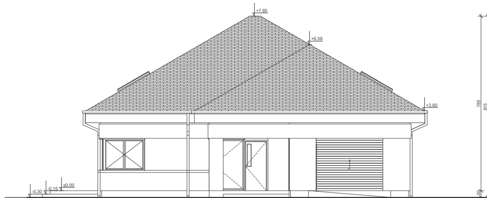
ELEWACJA FRONTOWA
