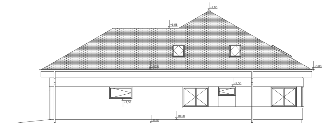
ELEWACJA BOK 2
