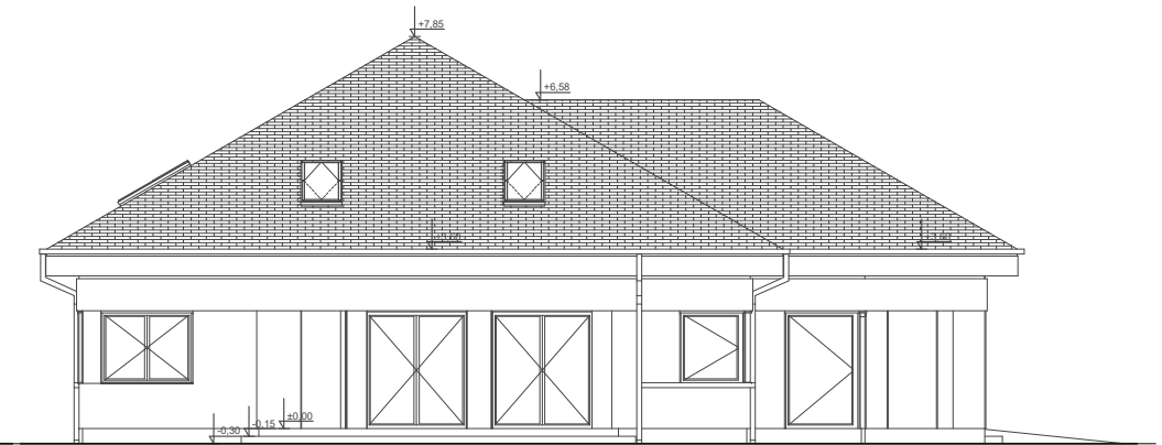
ELEWACJA BOK 1
