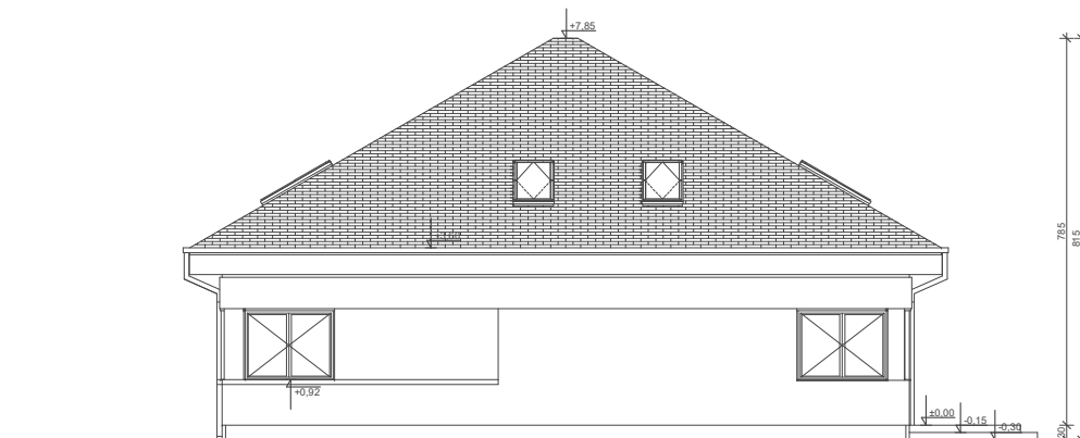
ELEWACJA OGRODOWA
