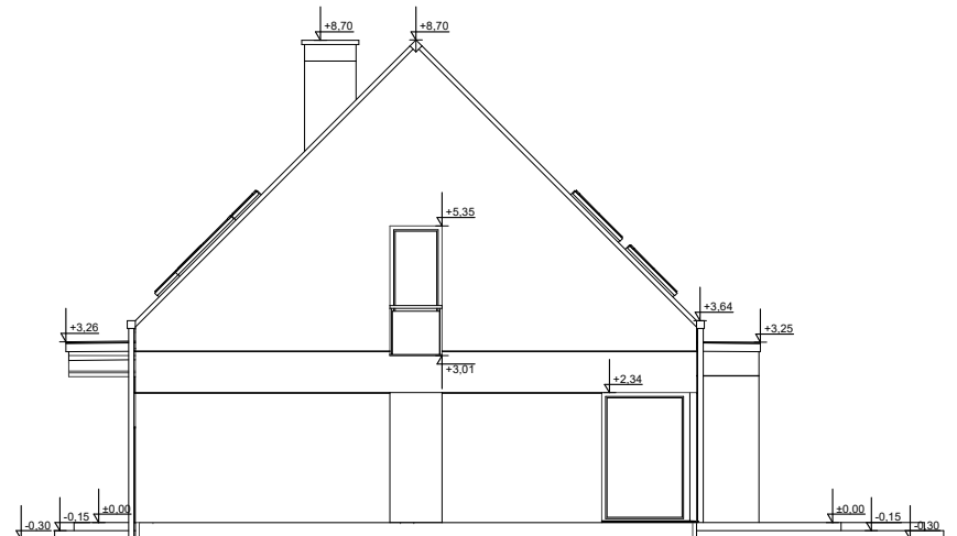
ELEWACJA BOK 2
