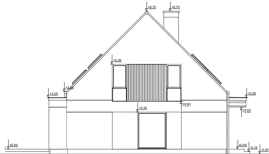
ELEWACJA BOK 1
