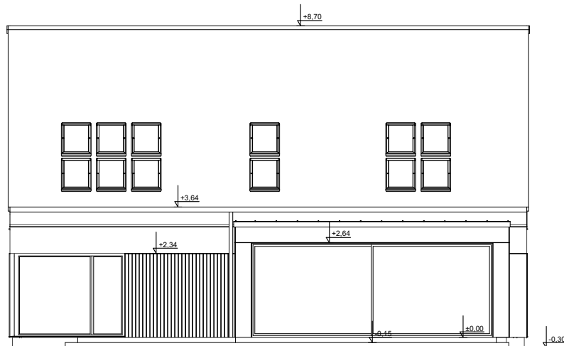
ELEWACJA OGRODOWA
