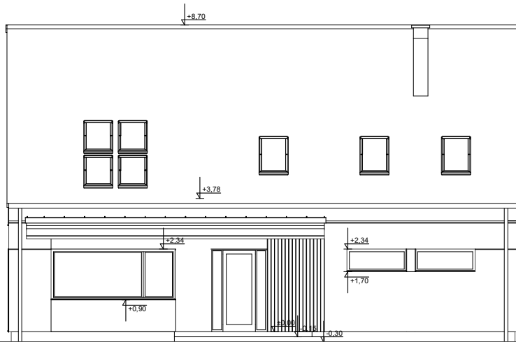
ELEWACJA FRONTOWA
