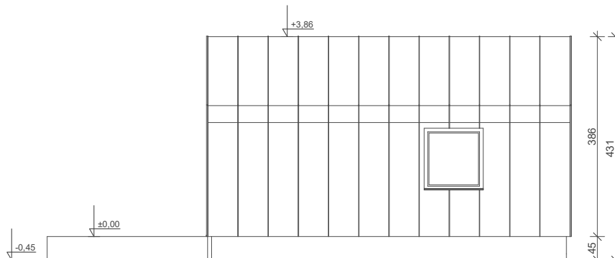
ELEWACJA OGRODOWA
