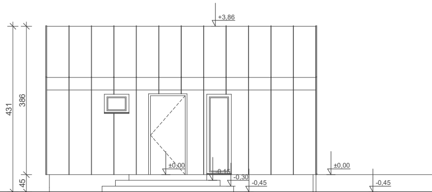
ELEWACJA FRONTOWA
