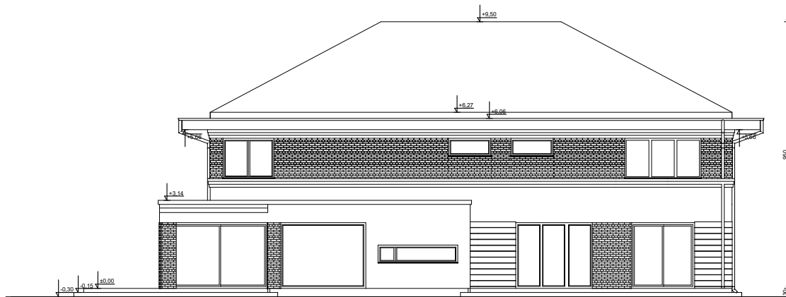
ELEWACJA OGRODOWA
