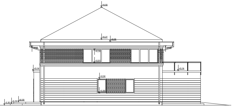
ELEWACJA BOK 1
