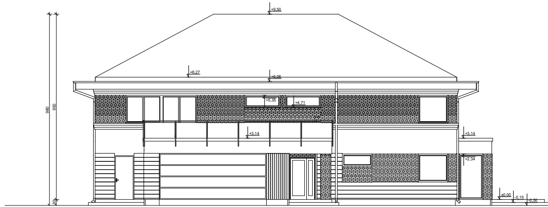
ELEWACJA FRONTOWA
