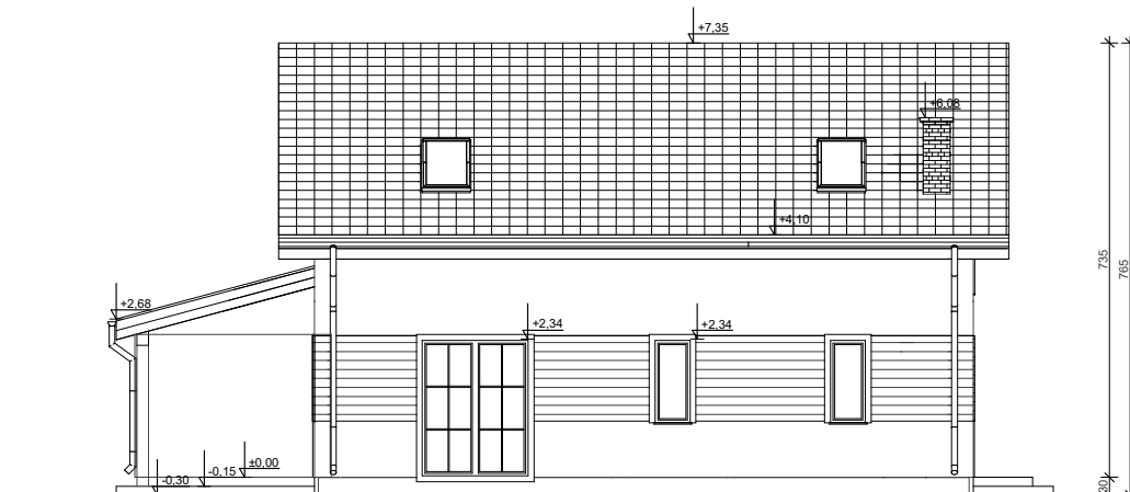
ELEWACJA OGRODOWA
