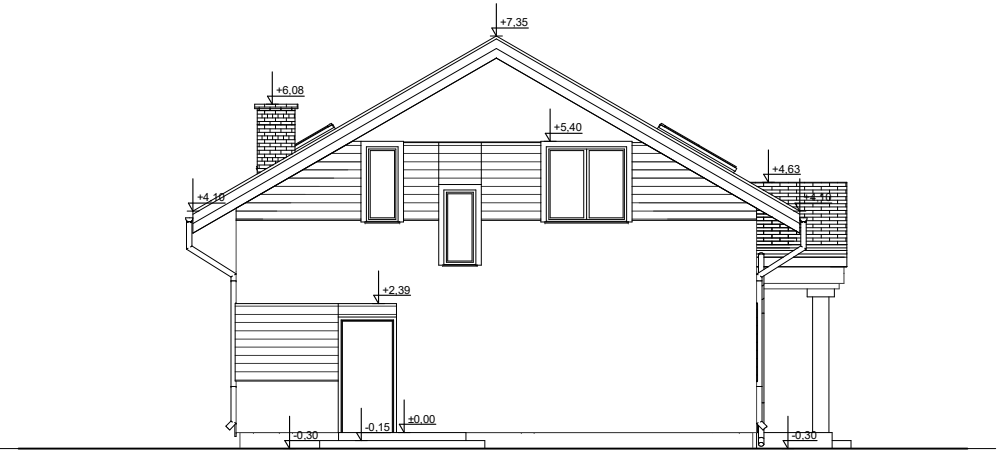
ELEWACJA BOK 1
