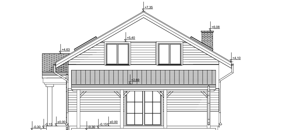
ELEWACJA BOK 2
