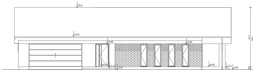
ELEWACJA FRONTOWA
