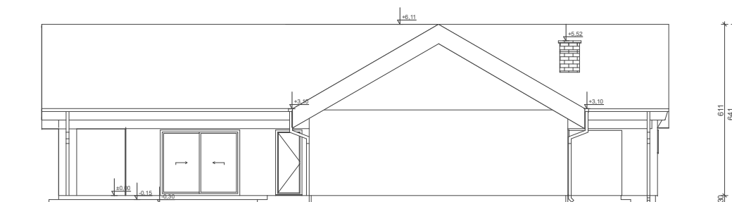
ELEWACJA OGRODOWA
