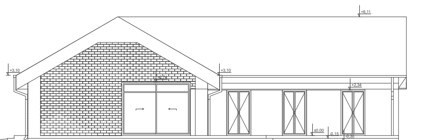
ELEWACJA BOK 2
