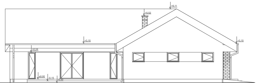
ELEWACJA BOK 1
