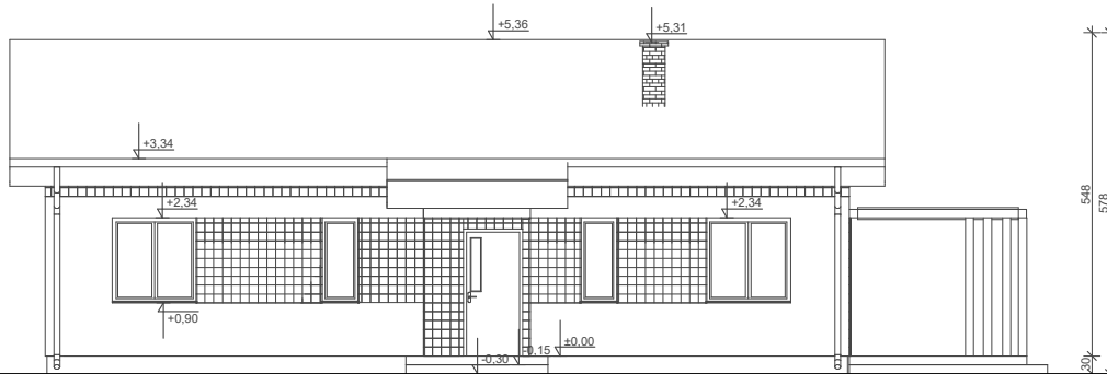
ELEWACJA FRONTOWA
