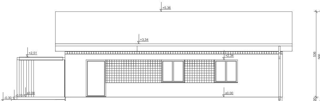
ELEWACJA OGRODOWA
