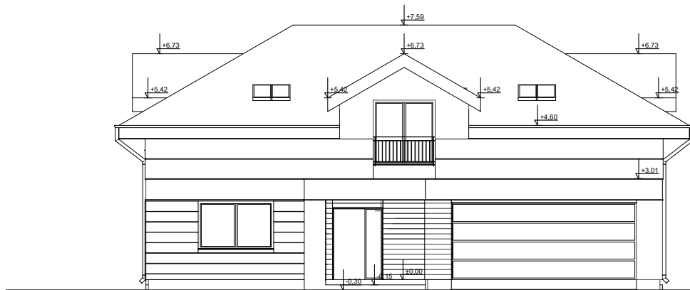
ELEWACJA FRONTOWA
