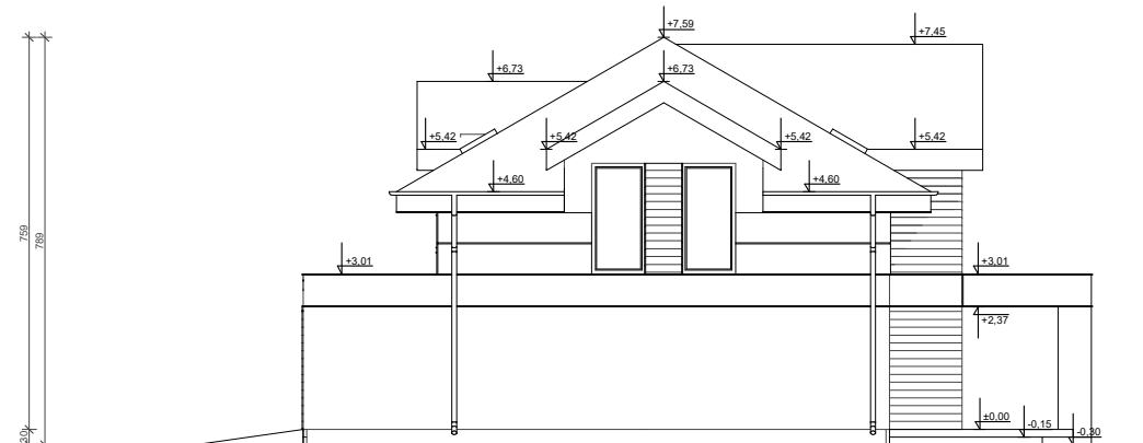
ELEWACJA BOK 2
