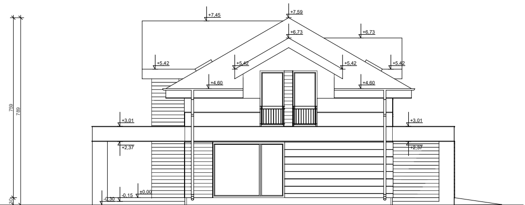
ELEWACJA BOK 1
