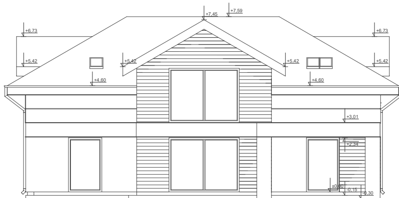
ELEWACJA OGRODOWA
