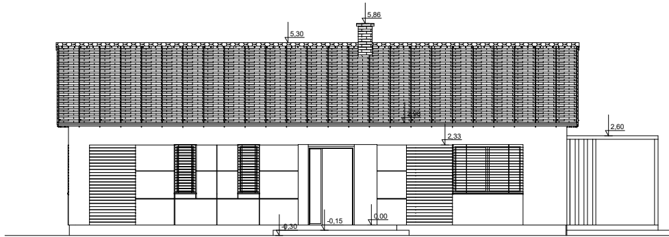
ELEWACJA FRONTOWA
