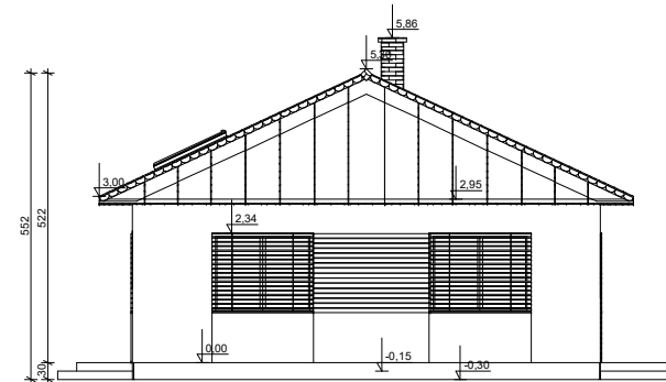
ELEWACJA BOK 1
