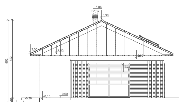
ELEWACJA BOK 2
