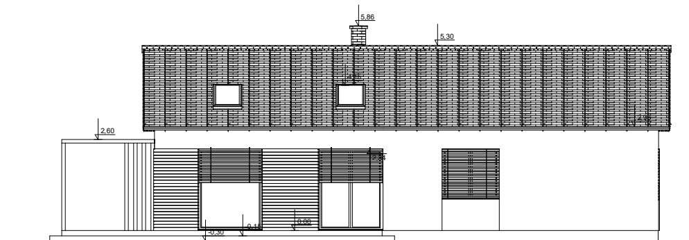
ELEWACJA OGRODOWA
