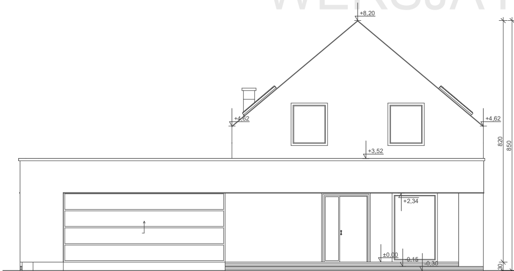
ELEWACJA FRONTOWA
