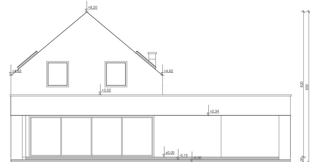
ELEWACJA OGRODOWA
