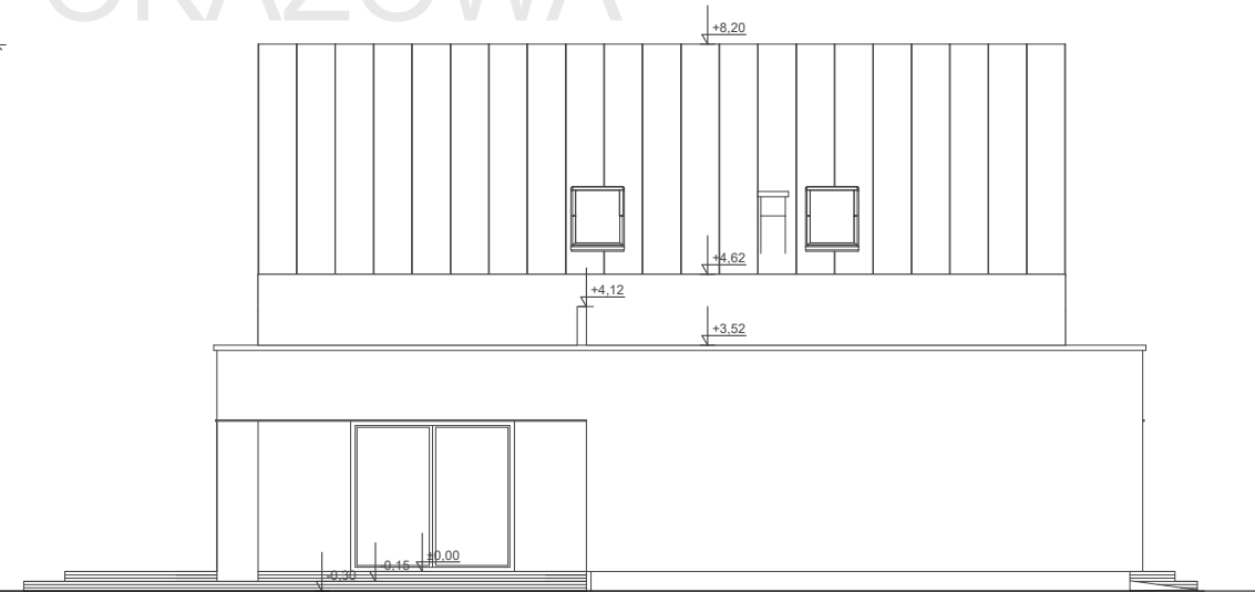
ELEWACJA BOK 1
