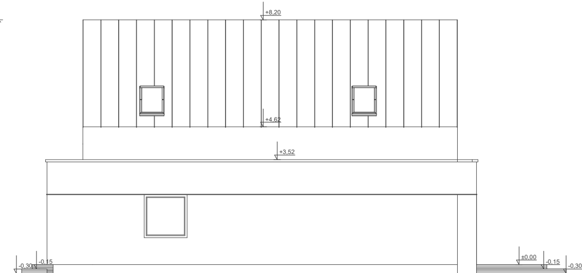
ELEWACJA BOK 2
