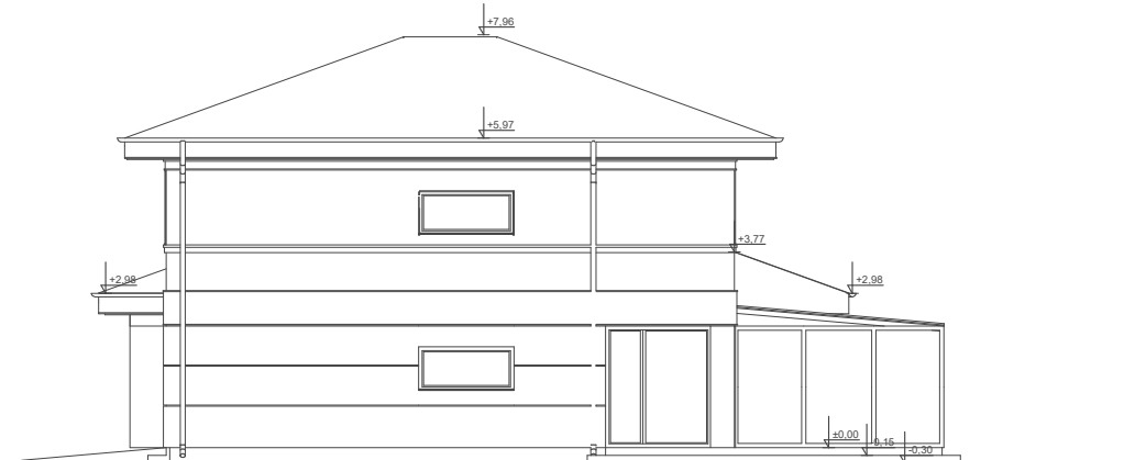
ELEWACJA BOK 2
