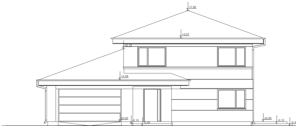
ELEWACJA FRONTOWA
