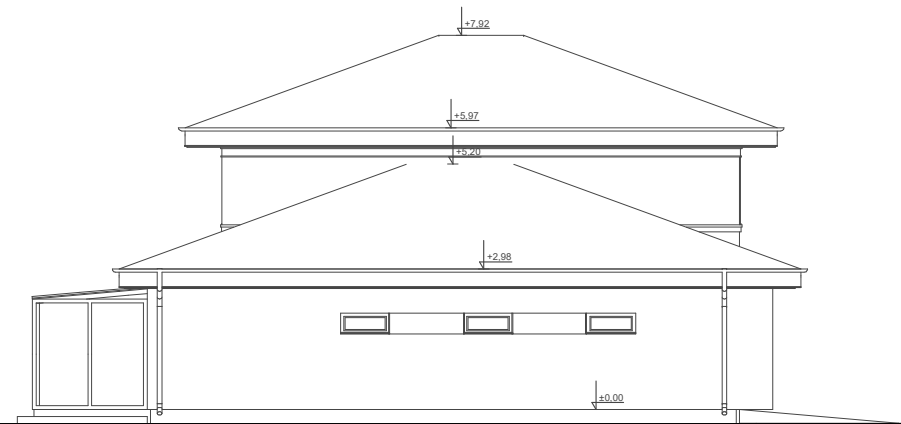
ELEWACJA BOK 1
