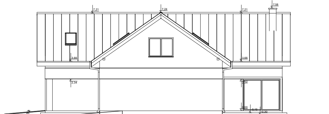
ELEWACJA BOK 2
