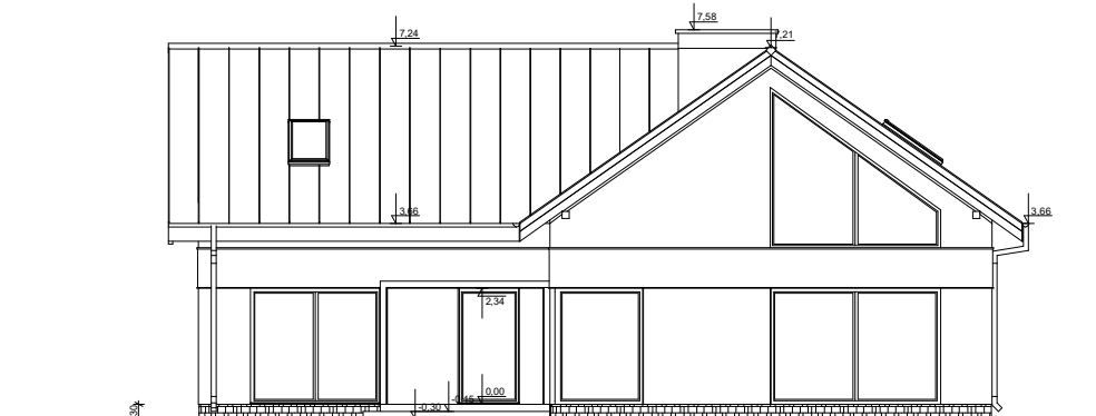
ELEWACJA OGRODOWA
