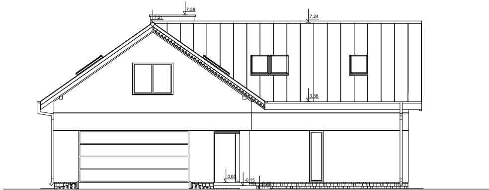
ELEWACJA FRONTOWA
