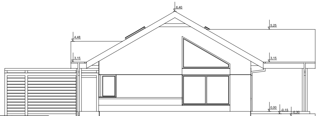
ELEWACJA BOK 2
