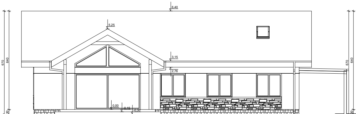
ELEWACJA OGRODOWA
