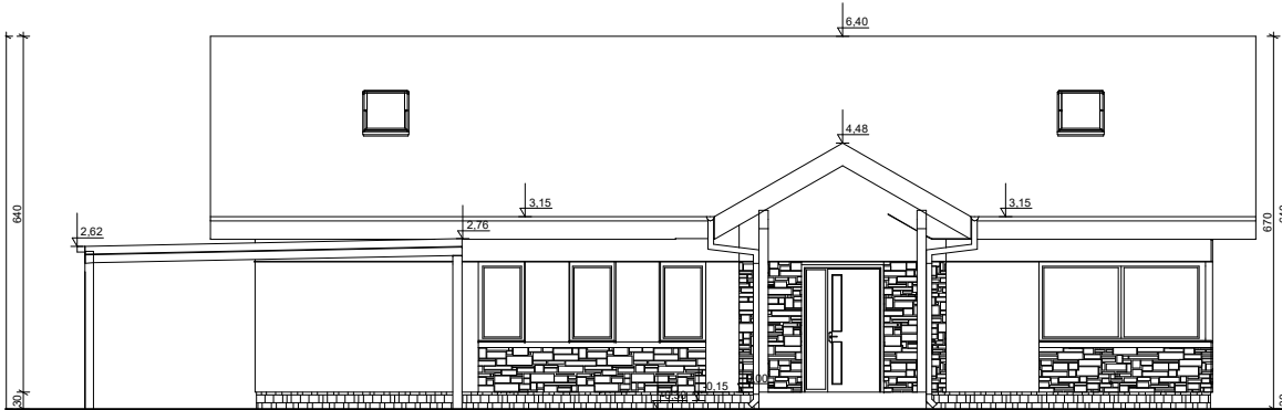
ELEWACJA FRONTOWA
