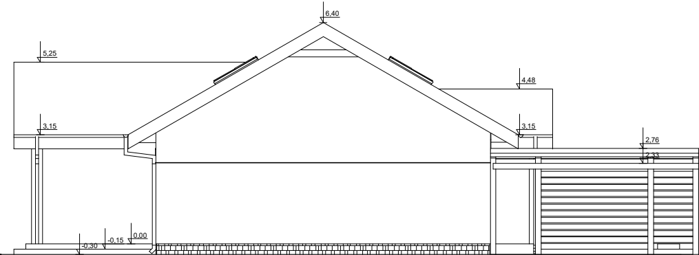
ELEWACJA BOK 1
