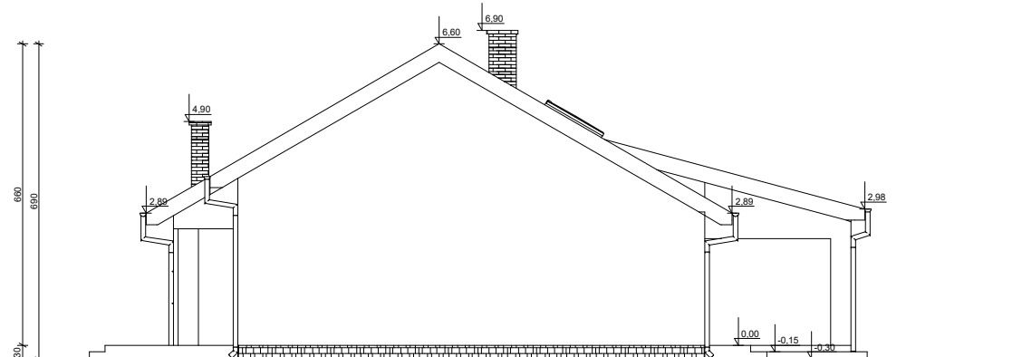
ELEWACJA BOK 2
