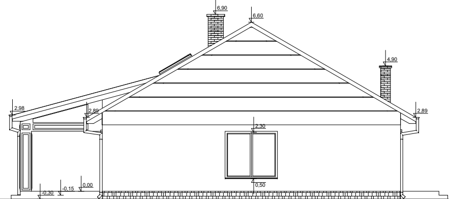
ELEWACJA BOK 1
