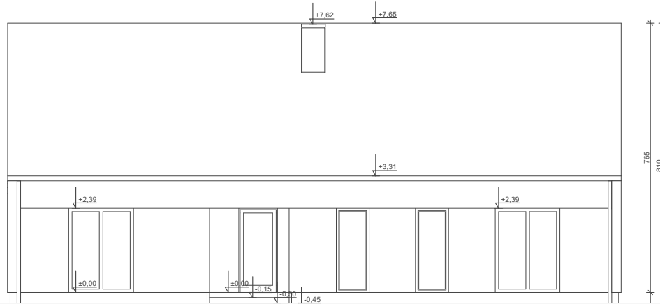
ELEWACJA FRONTOWA
