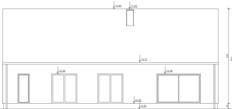
ELEWACJA OGRODOWA
