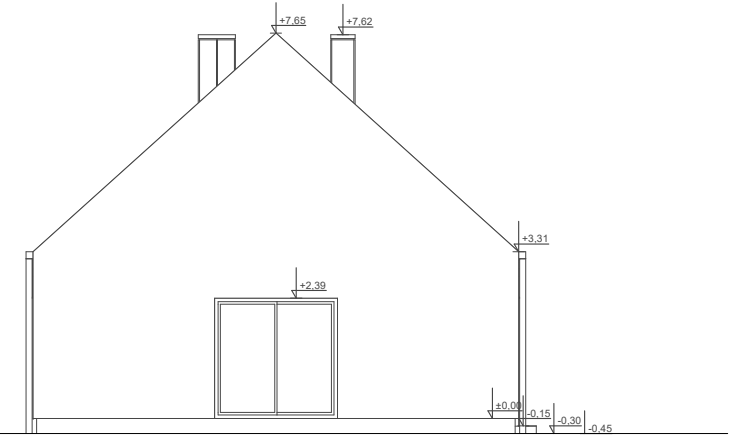
ELEWACJA BOK 1
