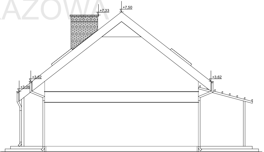
ELEWACJA BOK 1
