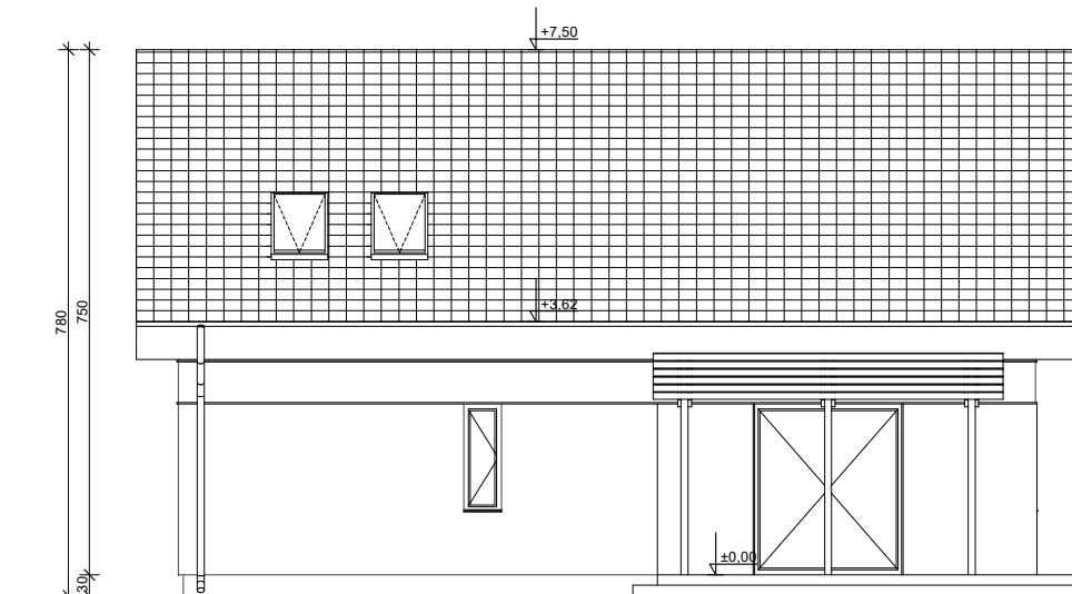
ELEWACJA OGRODOWA
