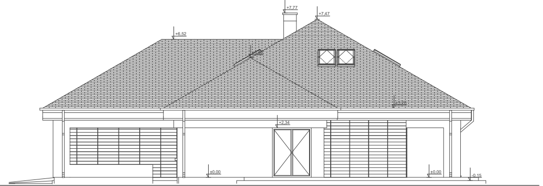
ELEWACJA BOK 1
