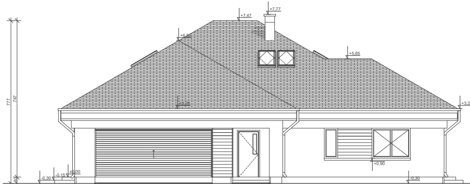
ELEWACJA FRONTOWA
