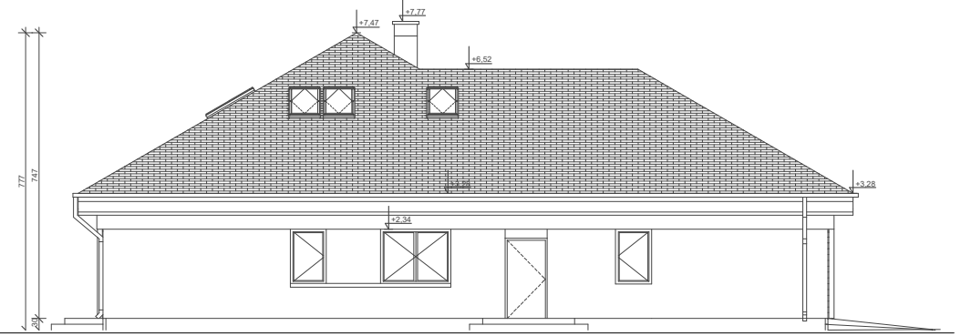
ELEWACJA BOK 2
