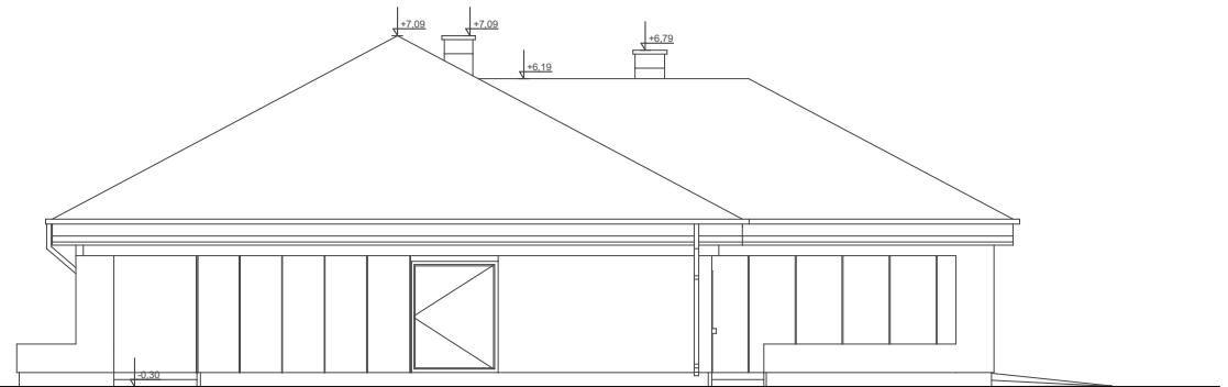
ELEWACJA BOK 2
