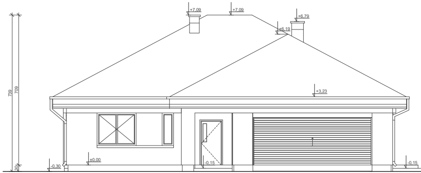
ELEWACJA FRONTOWA
