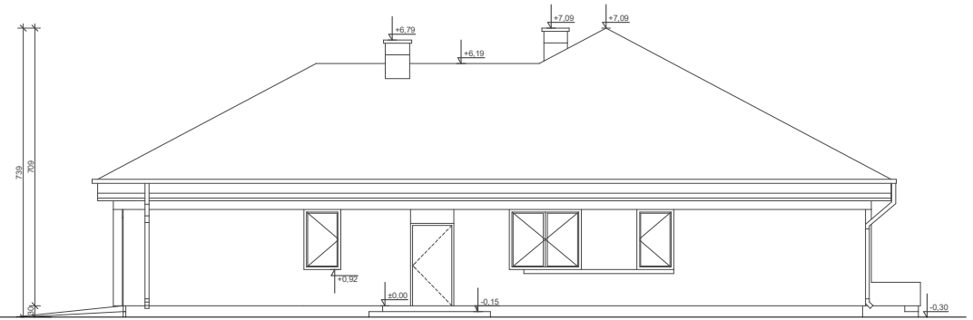
ELEWACJA BOK 1
