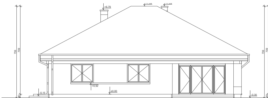
ELEWACJA OGRODOWA
