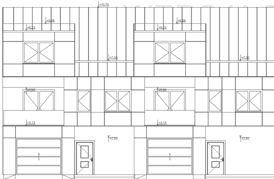
ELEWACJA WSCHODNIA
